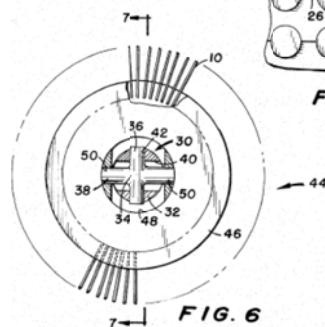
Рис. 4 – Фигуры маховика из патента университета Джона Хопкинса, автор Давид Рабенхорст 1972 г.
