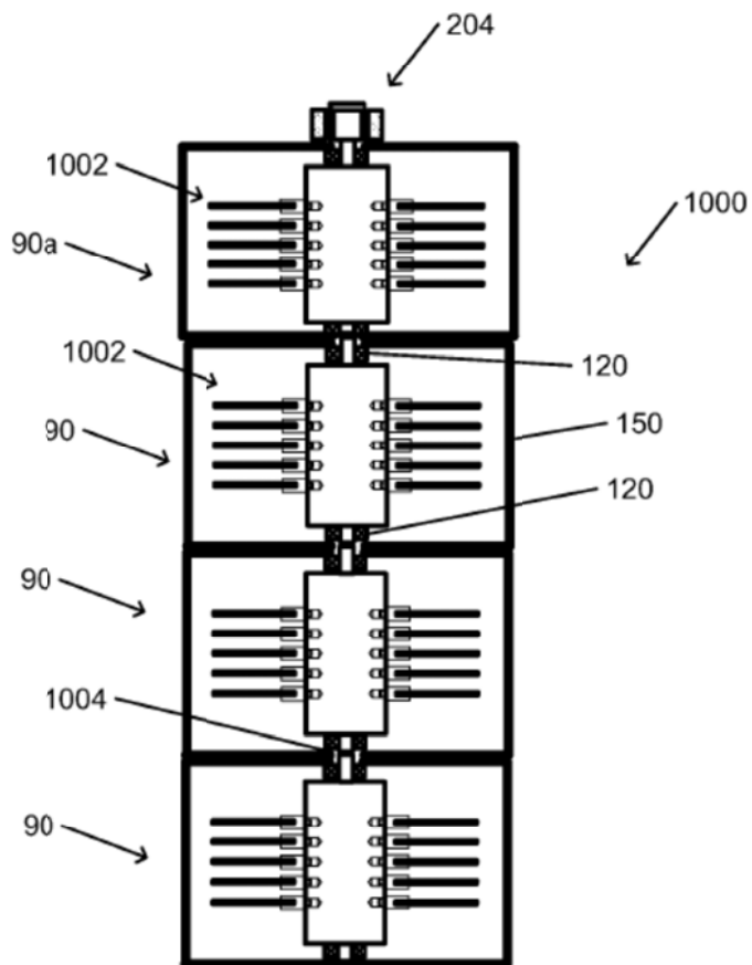
Рис. 3 – Фигуры маховика из патента фирмы «Чакратек» 2017 г.
